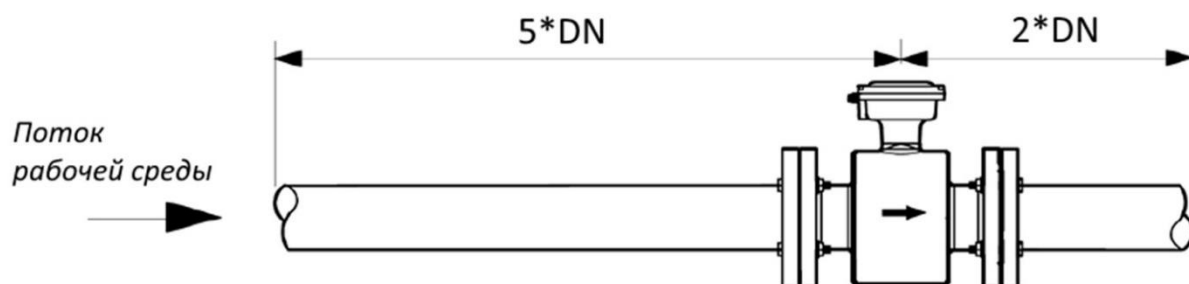
Рисунок 5 - Прямые участки
