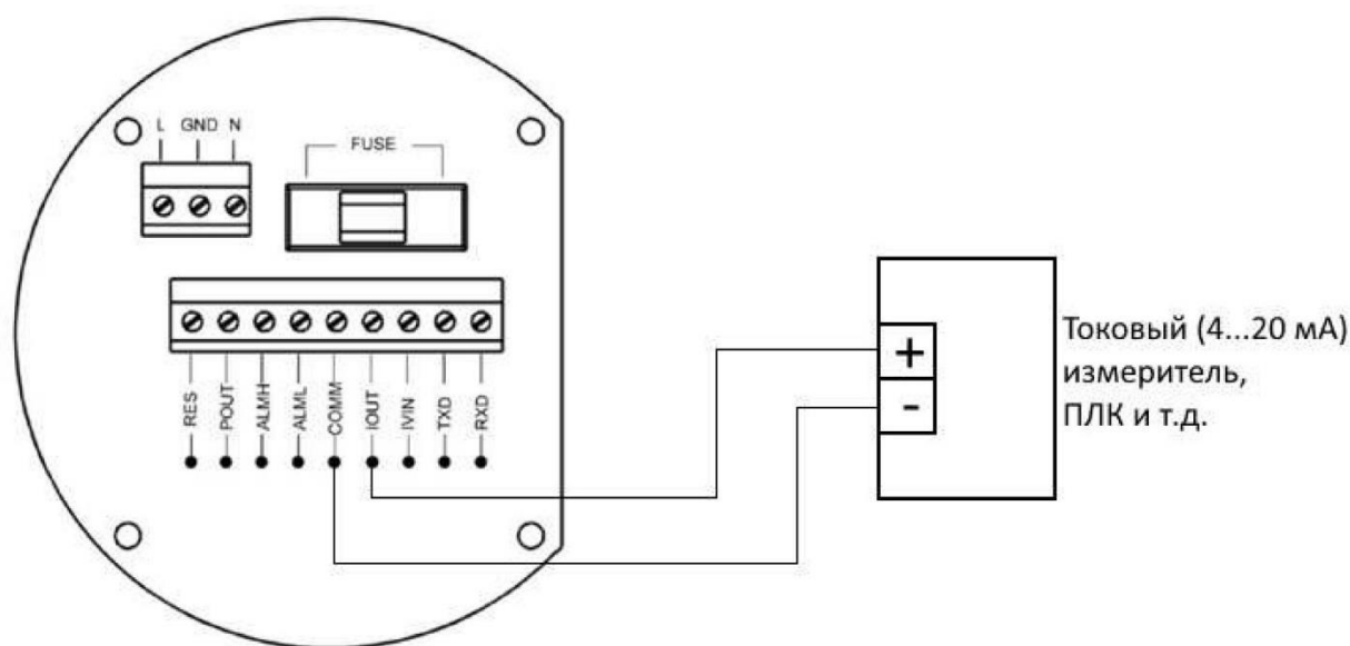
Рисунок 16 - Снятие сигнала 4...20 мА
