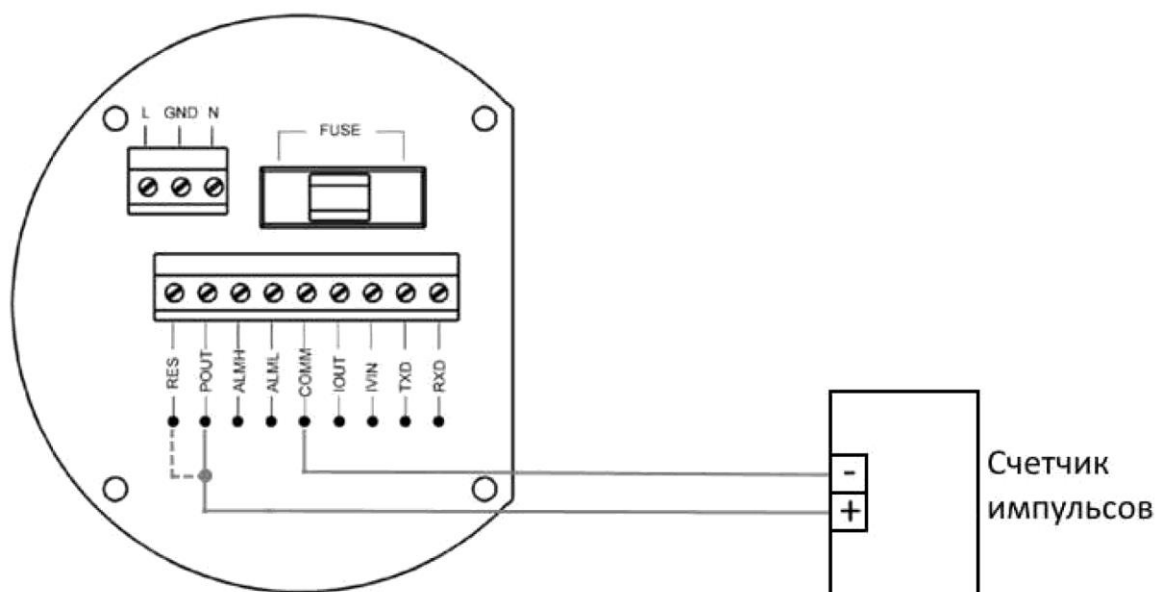
Рисунок 18 - Снятие импульсного или частотного сигнала с присутствием электромагнитного шума
