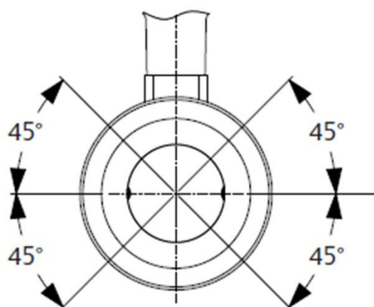
Рисунок 12 - Расположение электродов
