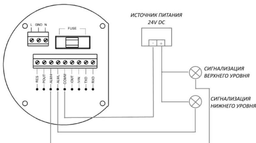
Рисунок 17 - Аварийная сигнализация
