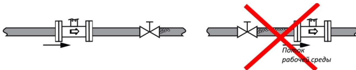
Рисунок 9 - Монтаж расходомера с трубопроводной арматурой
